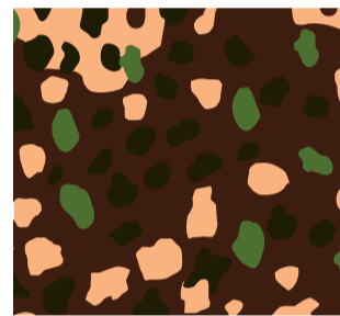
Dot Pea
